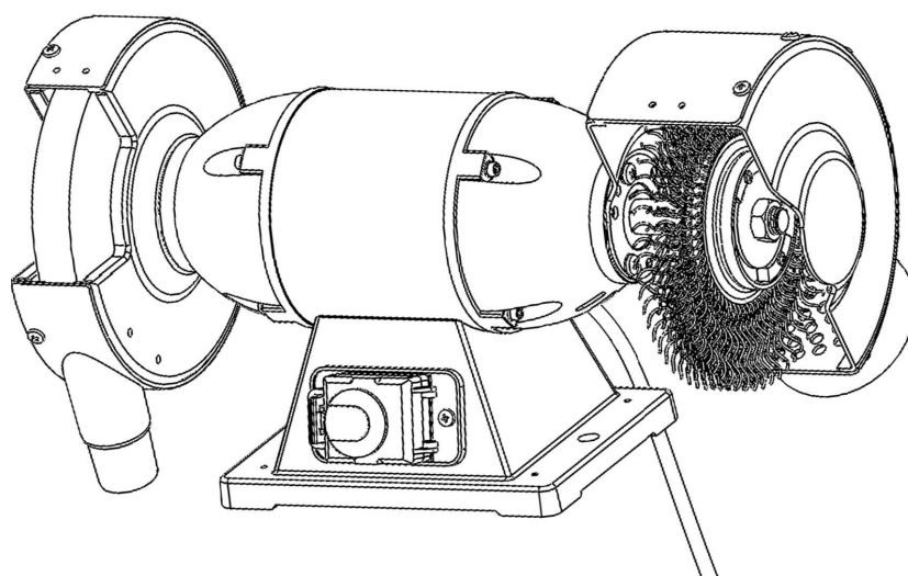
Schleifmaschine
