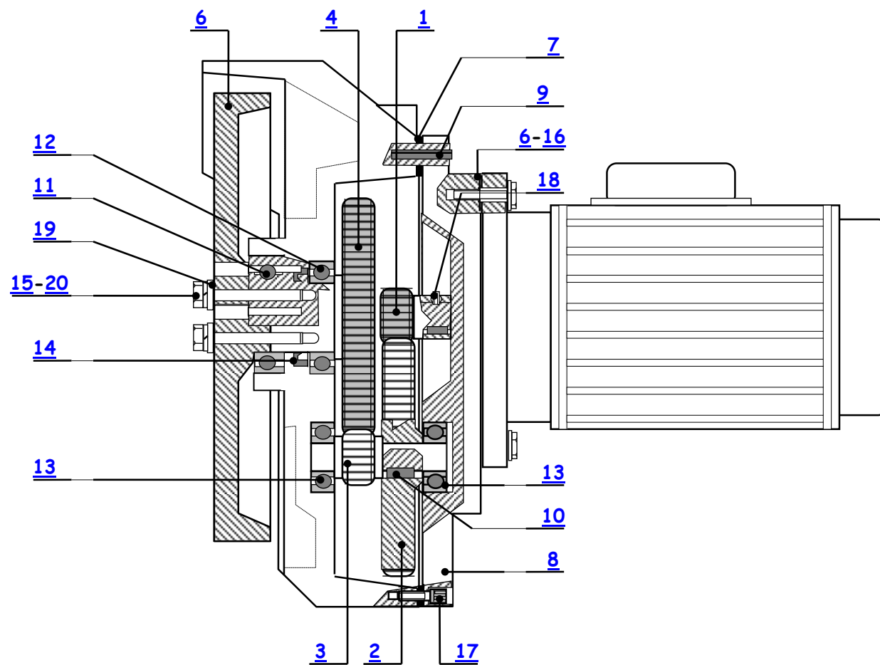
ENSEMBLE REDUCTEUR
