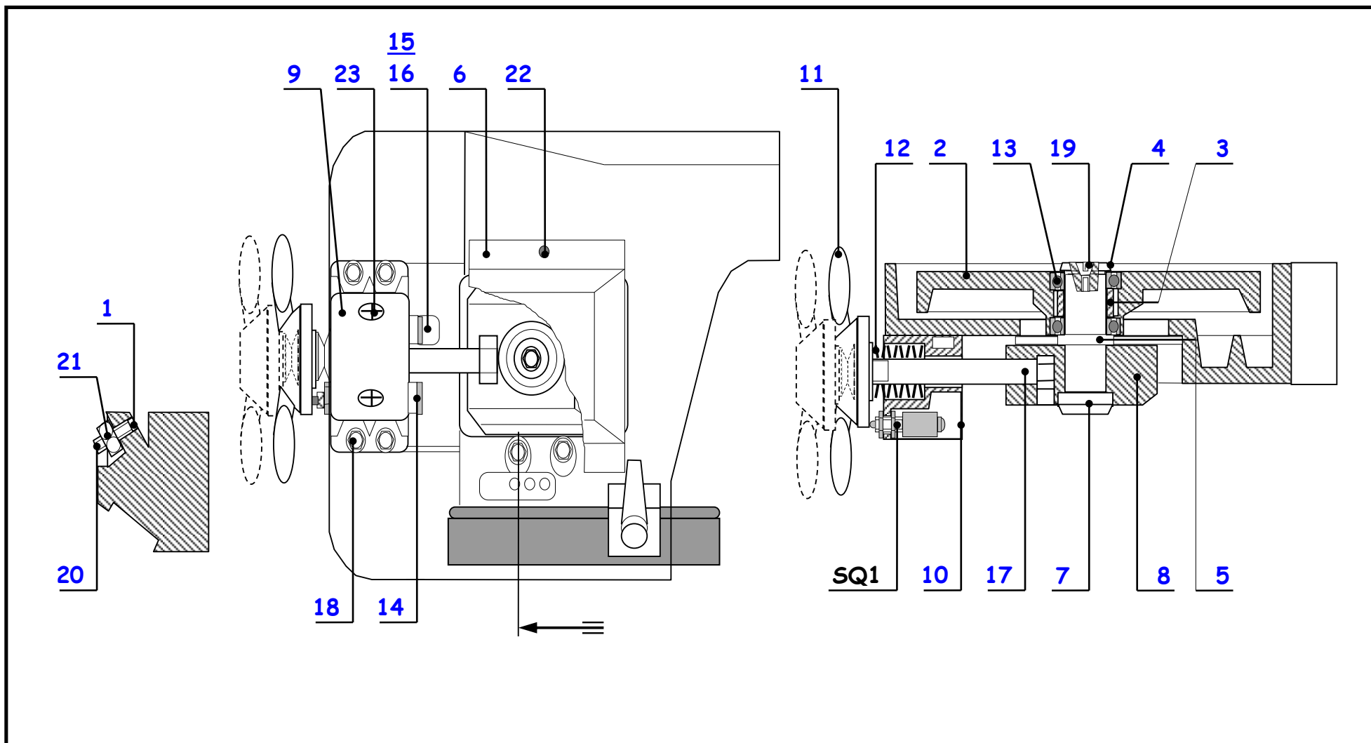
ENSAMBLE TENSION DE LAME
