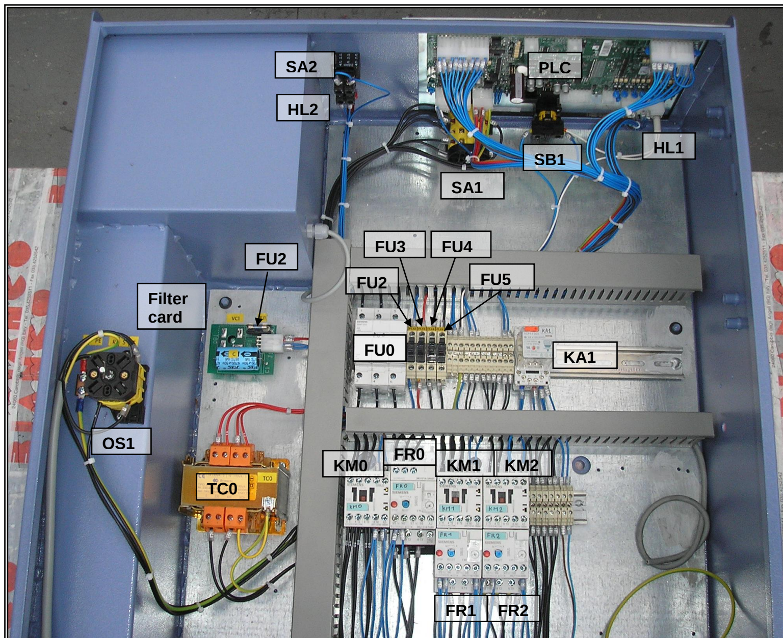
ARMOIRE ELECTRIQUE
