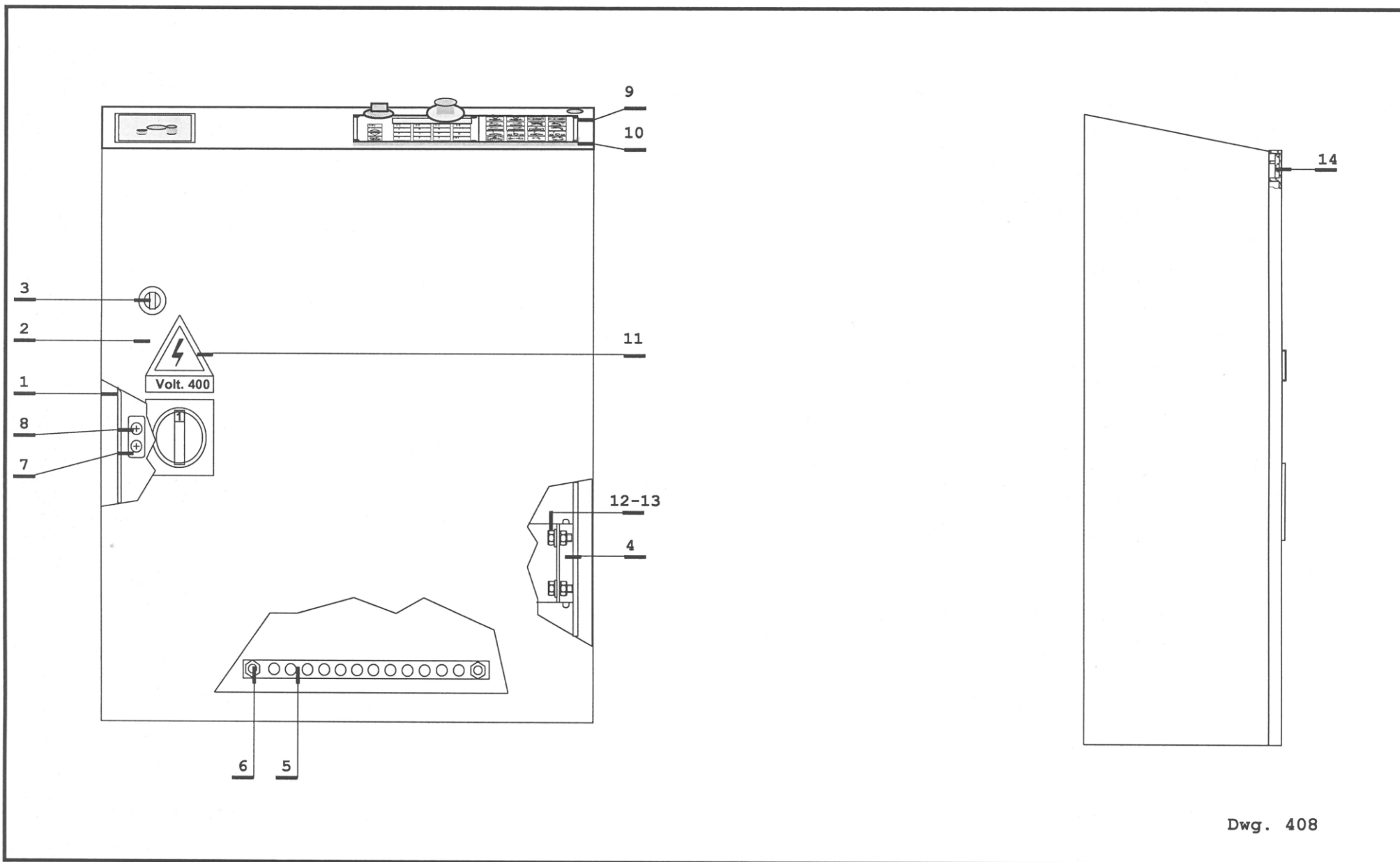
ARMOIRE ELECTRIQUE
