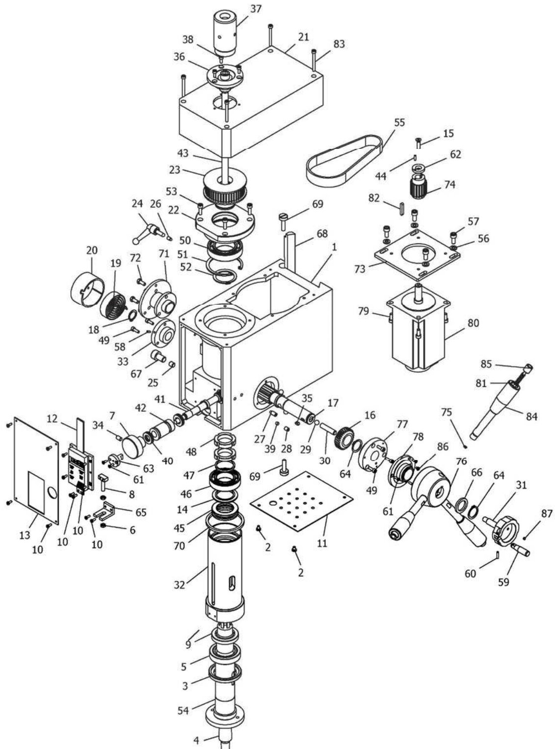
PBM-1839BDV Explosionszeichnung - 1
