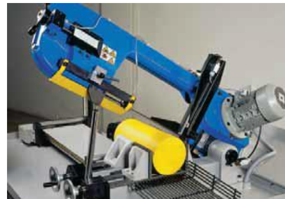
Etaux de serrage et d'avance- barre positionnés de part et d'autre du ruban
