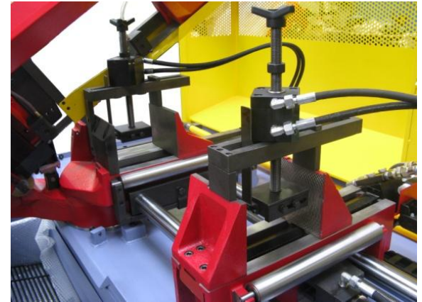
Dispositif de serrage vertical hydraulique pour coupes en paquets Capacités maxi : 200x130 mm
