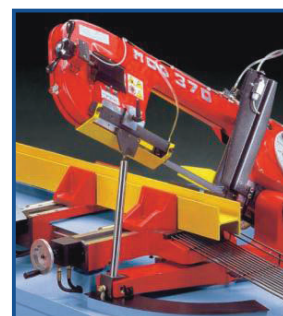
Vérin en tête d'archet Modèle A60°
