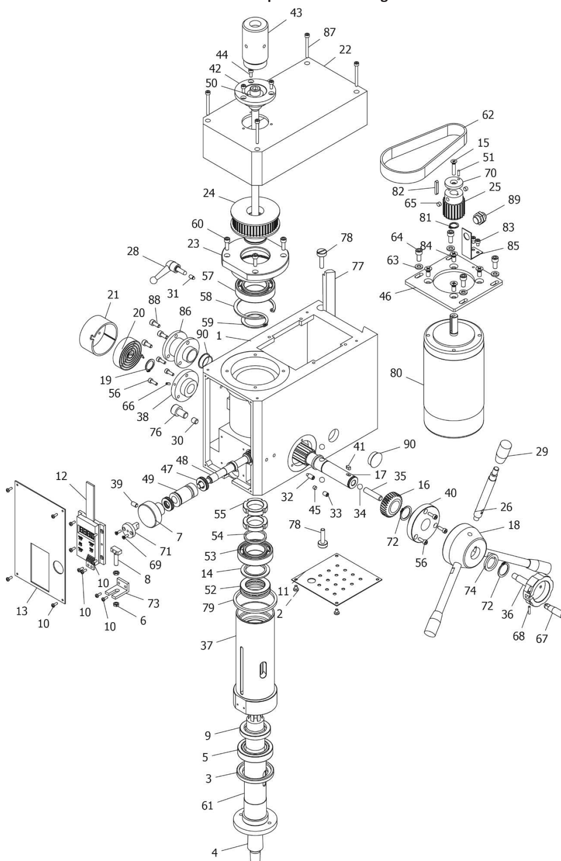
PBM-1839V Explosionszeichnung - 1
