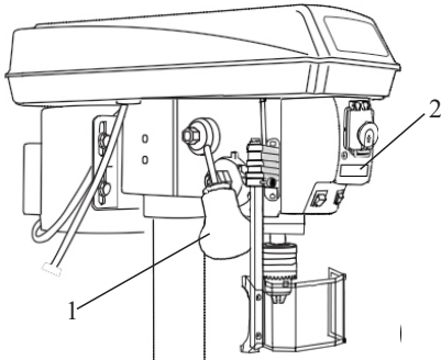
Variation mécanique de la vitesse (Fig. 24) Il s'agit d'une perceuse d'établi à vitesse variable. Pour
